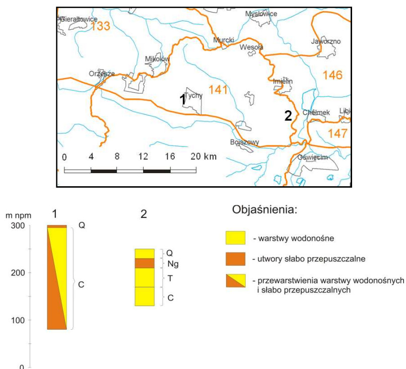
Rysunek 96. Profile geologiczne i ich lokalizacja w JCWPd nr 141
