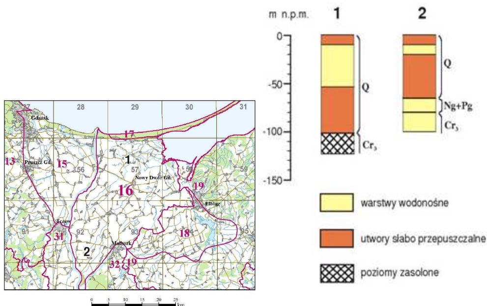
Rysunek 32. Profile geologiczne i ich lokalizacja w JCWPd nr 16. Źródło: PSH
