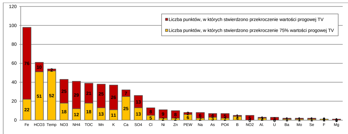
Rysunek 19. Analiza wskaźników w odniesieniu do wartości progowej stanu dobrego oraz 75% wartości progowej stanu dobrego
