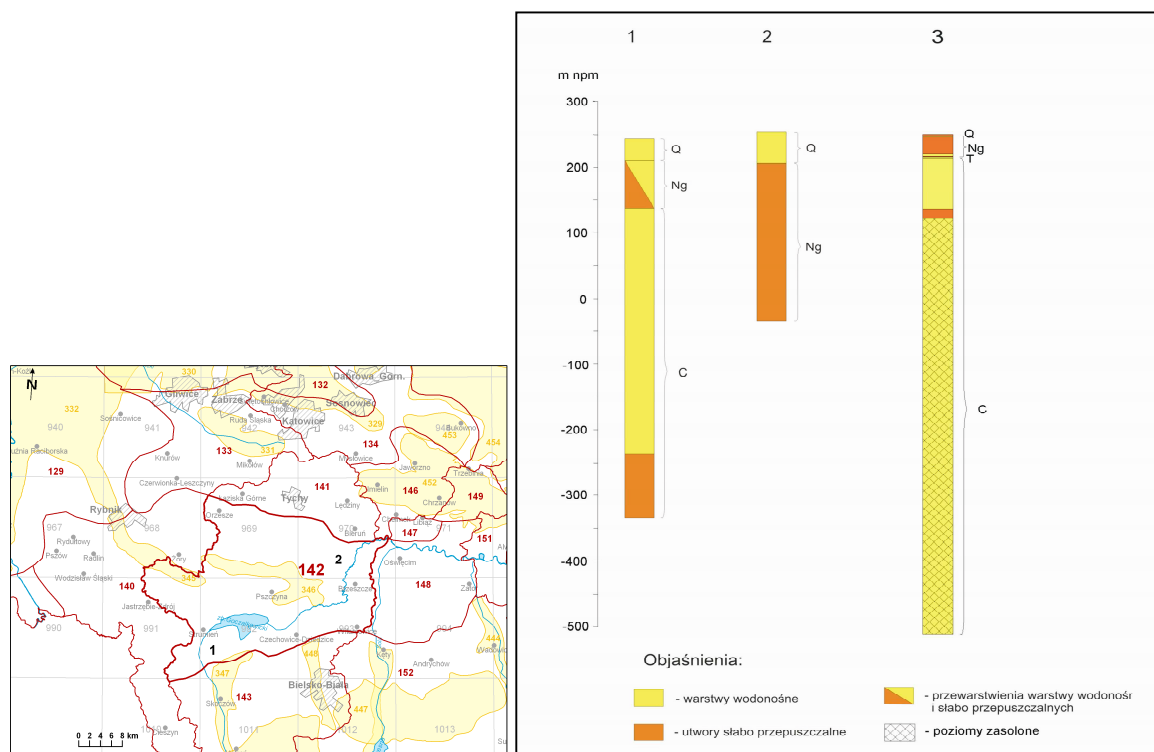
Rysunek 98. Profile geologiczne i ich lokalizacja w JCWPd nr 142. Źródło PSH
