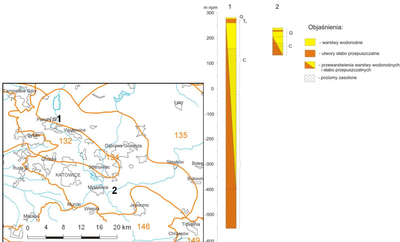
Rysunek 93. Profile geologiczne i ich lokalizacja w JCWPd nr 134
