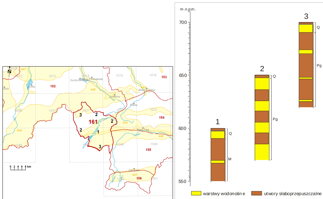
Rysunek 106. Profile geologiczne i ich lokalizacja w JCWPd nr 161. Źródło: PSH
