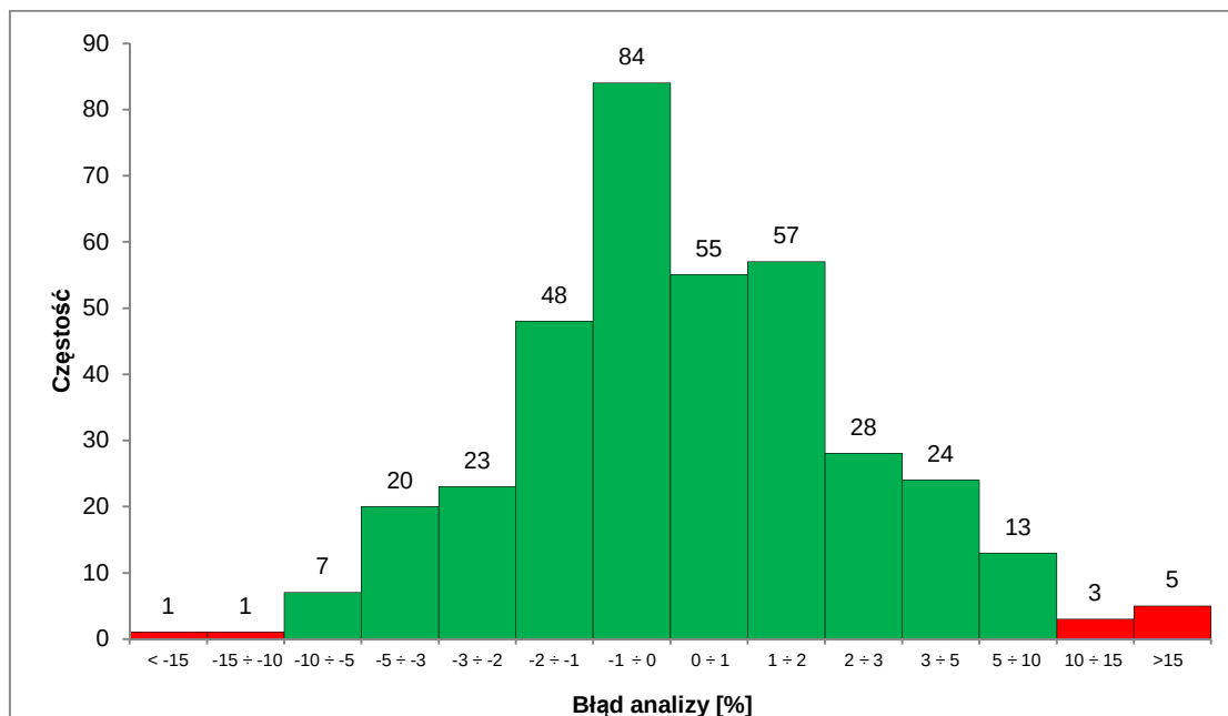
Rysunek 1. Rozkład błędu analizy na podstawie bilansu jonowego wody dla 370 analiz próbek wód podziemnych
