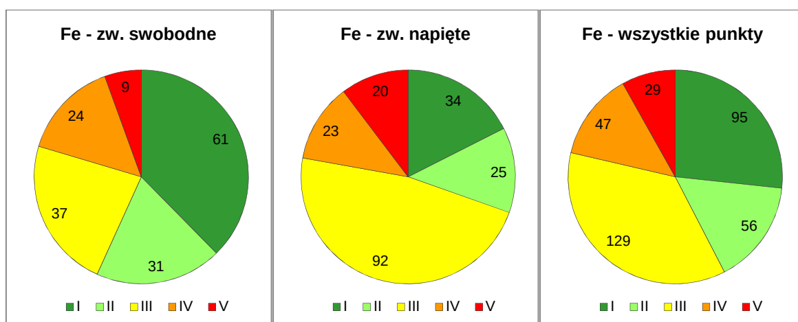
Rysunek 7. Klasy jakości wód podziemnych w 356 punktach pomiarowych wykorzystanych do oceny stanu chemicznego JCWPd wg danych z 2015 r., według wartości stężeń żelaza
