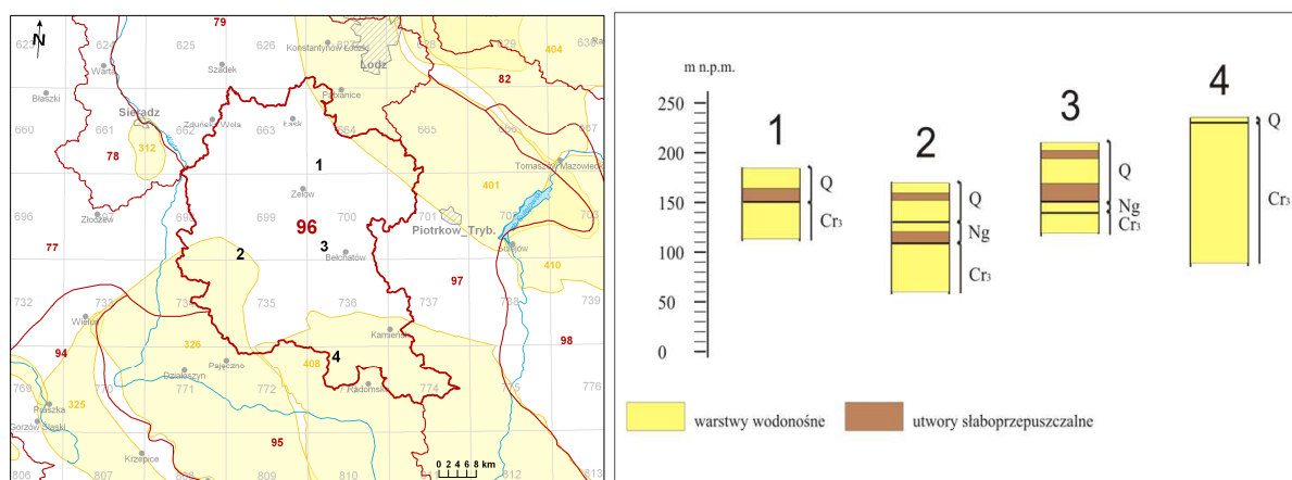
Rysunek 73. Profile geologiczne i ich lokalizacja w JCWPd nr 96
