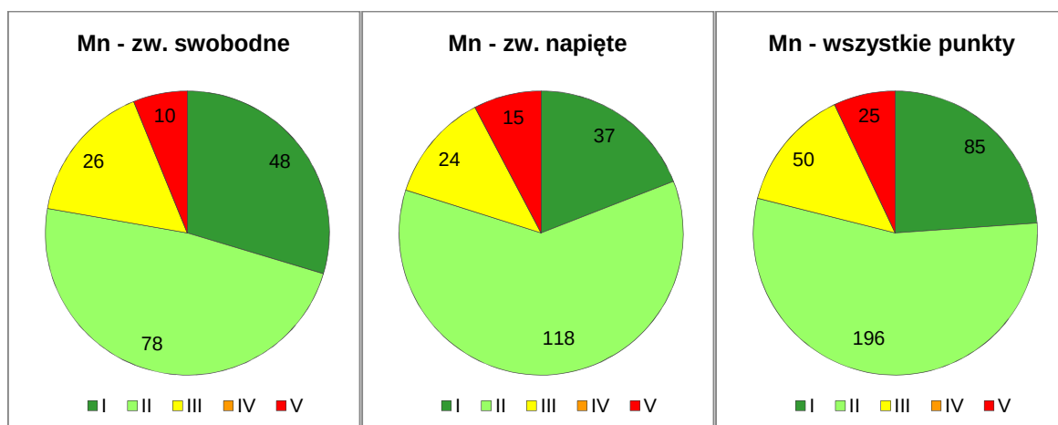
Rysunek 8. Klasy jakości wód podziemnych w 356 punktach pomiarowych wykorzystanych do oceny stanu chemicznego JCWPd wg danych z 2015 r., według wartości stężeń manganu
