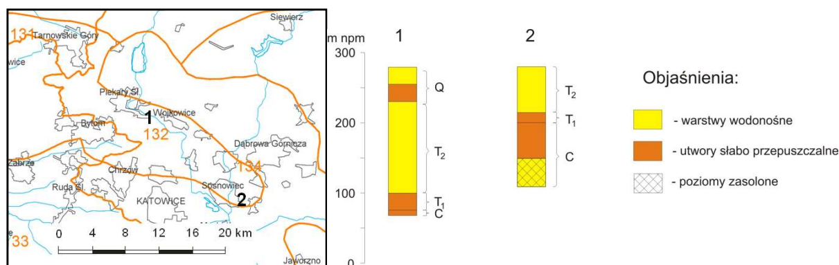
Rysunek 91. Profile geologiczne i ich lokalizacja w JCWPd nr 132
