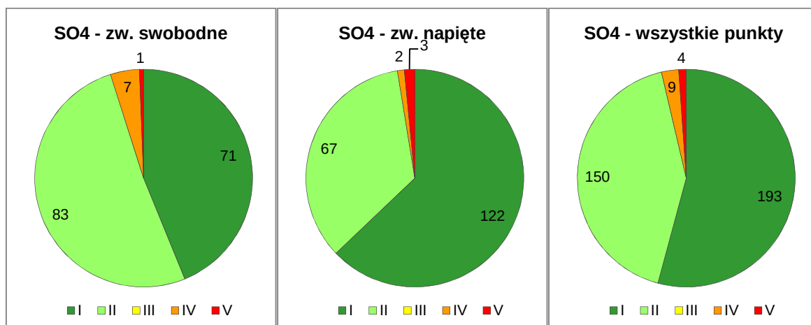
Rysunek 16. Klasy jakości wód podziemnych w 356 punktach pomiarowych wykorzystanych do oceny stanu chemicznego JCWPd wg danych z 2015 r., według wartości stężeń siarczanów
