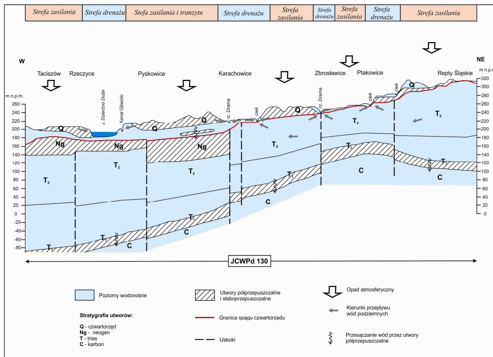
Rysunek 90. Model koncepcyjny krążenia wód podziemnych w JCWPd nr 130. Źródło: PSH
