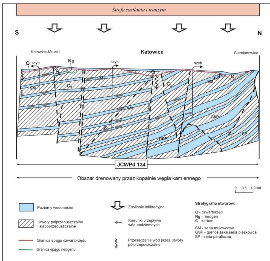
Rysunek 95. Model koncepcyjny krążenia wód podziemnych w JCWPd nr 134. Źródło: PSH
