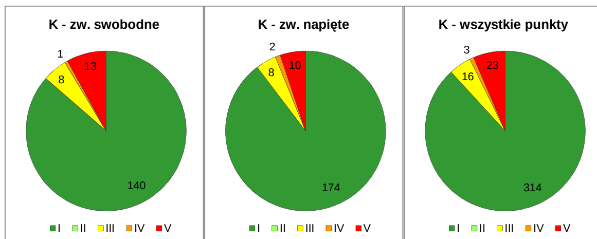
Rysunek 13. Klasy jakości wód podziemnych w 356 punktach pomiarowych wykorzystanych do oceny stanu chemicznego JCWPd wg danych z 2015 r., według wartości stężeń potasu
