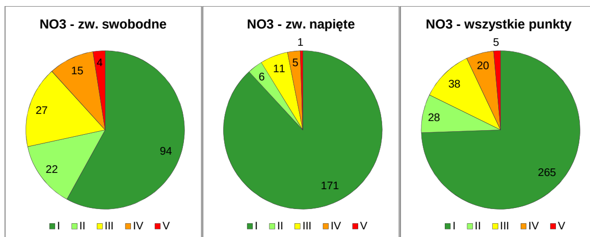
Rysunek 20. Klasy jakości wód podziemnych wg RMŚ z 21 grudnia 2015, w 356 punktach pomiarowych wykorzystanych do oceny stanu chemicznego JCWPd wg danych z 2015 r., według wartości stężeń azotanów
