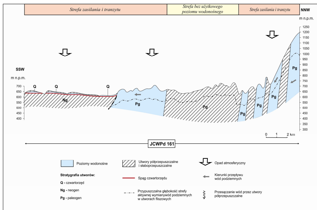
Rysunek 107. Model koncepcyjny krążenia wód podziemnych w JCWPd nr 161. Źródło: PSH
