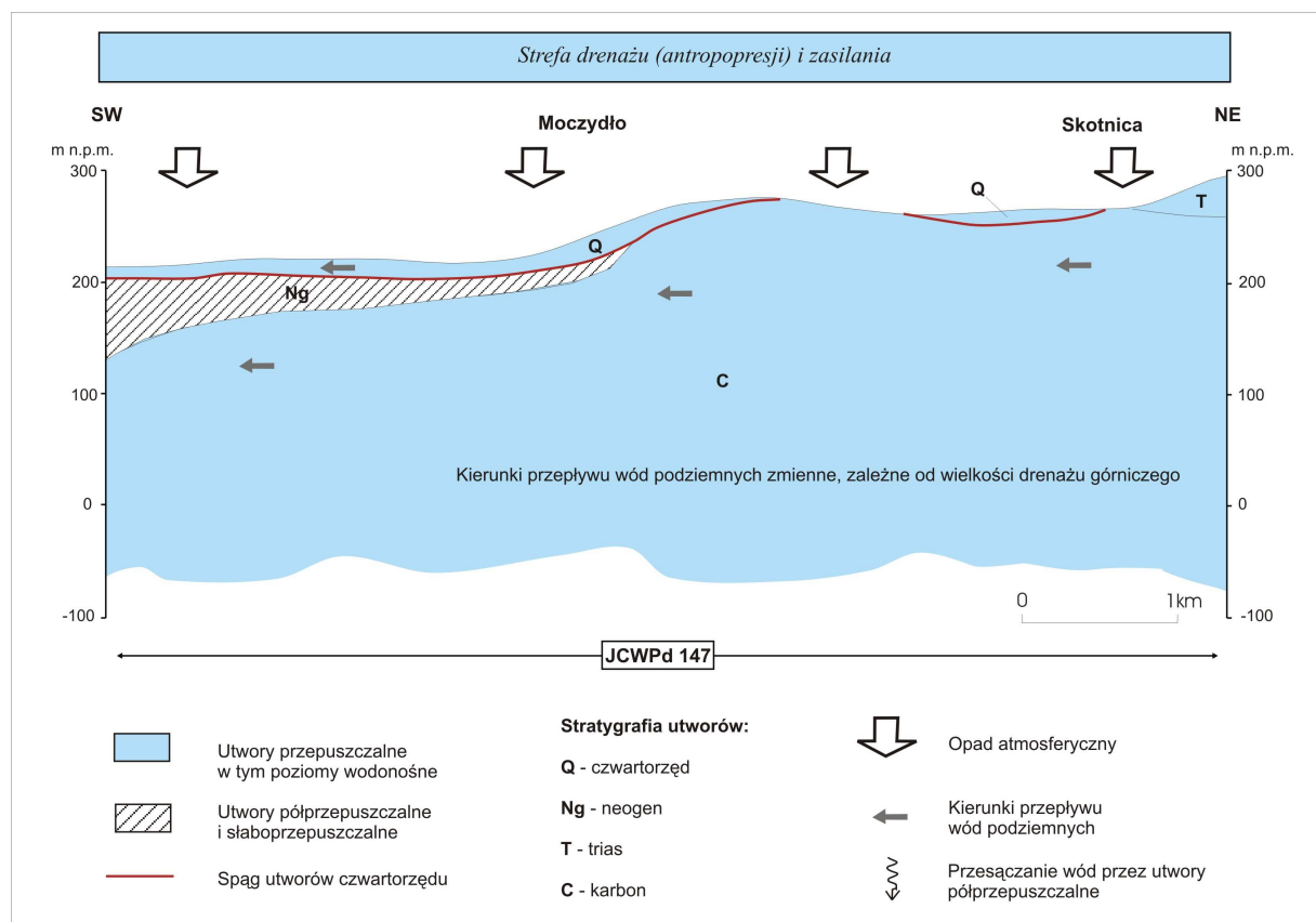
Rysunek 103. Schemat przepływu wód podziemnych w JCWPd nr 147. Źródło PSH
