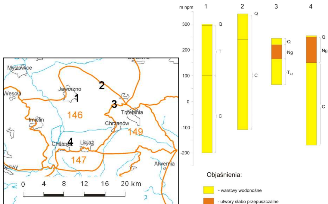
Rysunek 100. Profile geologiczne i ich lokalizacja w JCWPd nr 146
