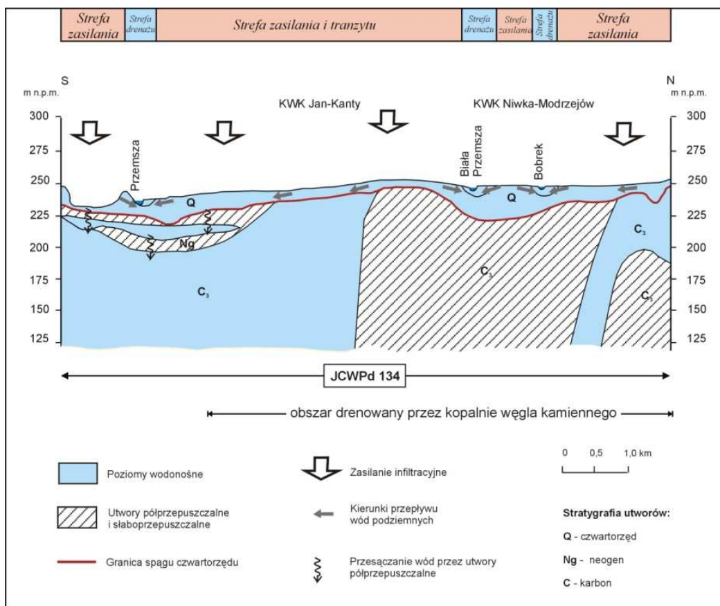
Rysunek 94. Model koncepcyjny krążenia wód podziemnych w JCWPd nr 134. Źródło: PSH
