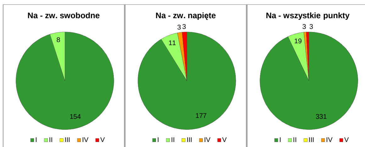
Rysunek 14. Klasy jakości wód podziemnych w 356 punktach pomiarowych wykorzystanych do oceny stanu chemicznego JCWPd wg danych z 2015 r., według wartości stężeń sodu
