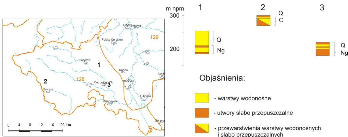
Rysunek 87. Profile geologiczne i ich lokalizacja w JCWPd nr 128
