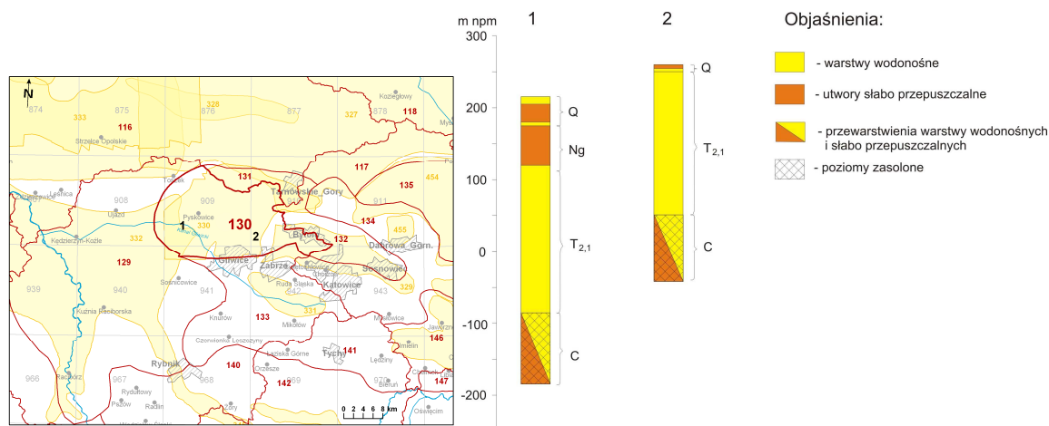
Rysunek 89. Profile geologiczne i ich lokalizacja w obrębie JCWPd nr 130. Źródło: PSH
