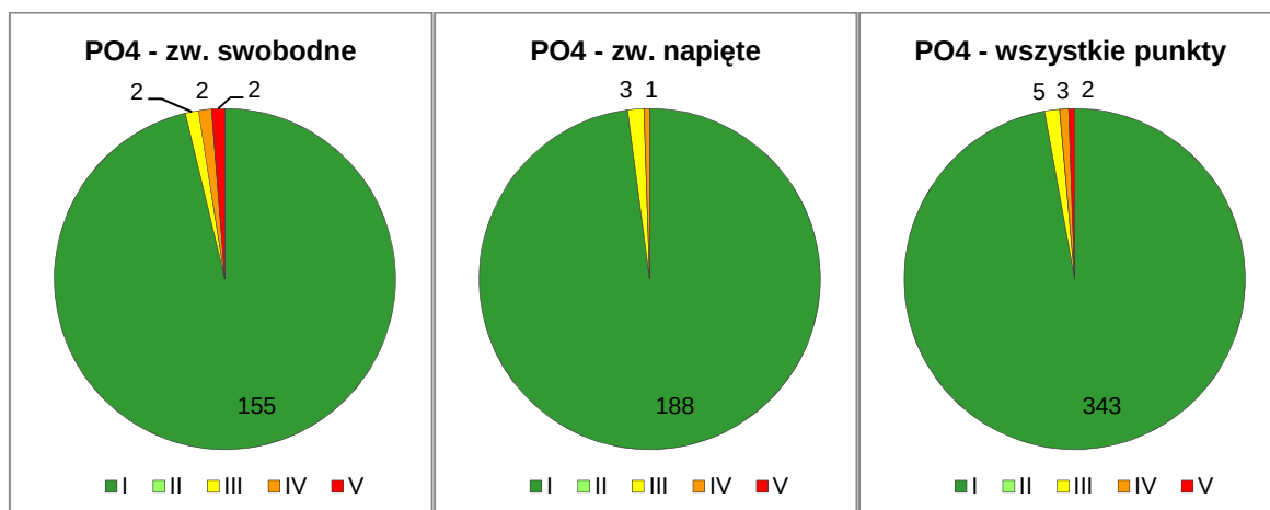
Rysunek 12. Klasy jakości wód podziemnych w 356 punktach pomiarowych wykorzystanych do oceny stanu chemicznego JCWPd wg danych z 2015 r., według wartości stężeń fosforanów
