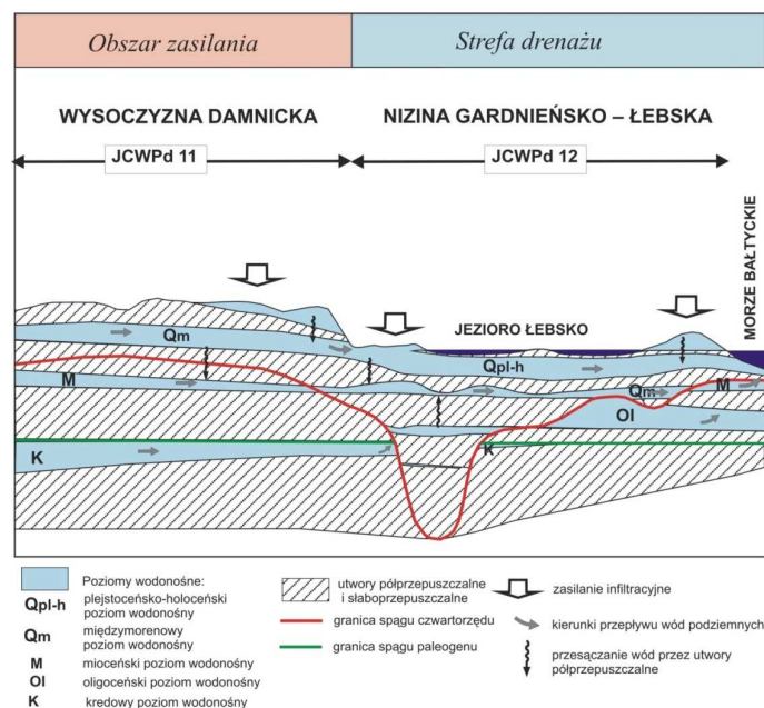
Rysunek 27. Model koncepcyjny krążenia wód podziemnych w JCWPd nr 12. Źródło: PSH
