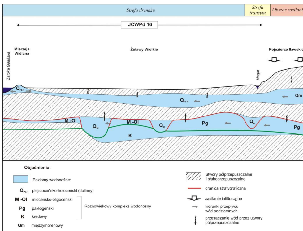
Rysunek 33. Model koncepcyjny krążenia wód podziemnych w JCWPd nr 16. Źródło: PSH
