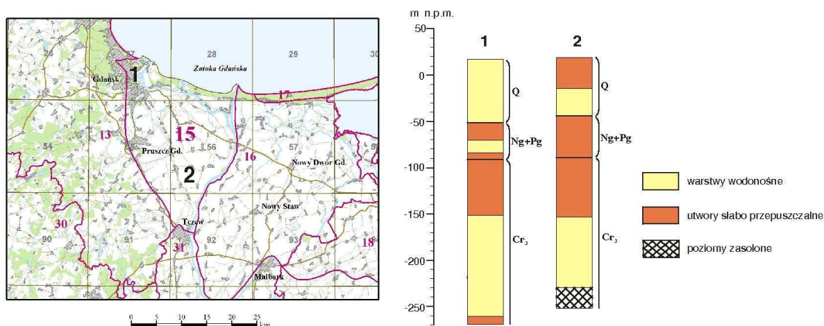
Rysunek 30. Profile geologiczne i ich lokalizacja w JCWPd nr 15. Źródło: PSH
