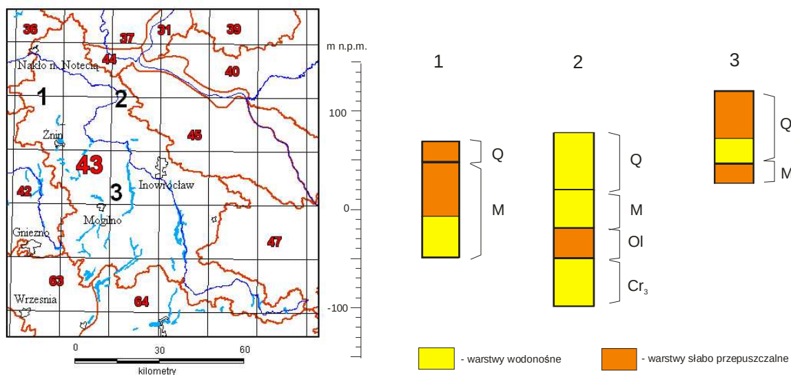
Rysunek 47. Profile geologiczne i ich lokalizacja w JCWPd nr 43
