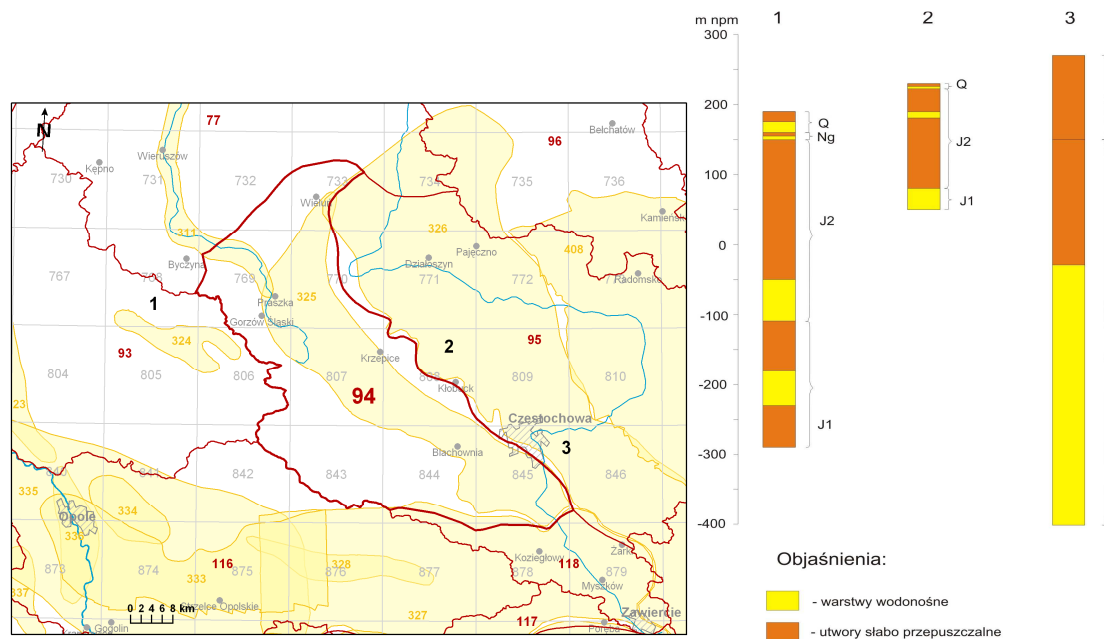
Rysunek 71. Profile geologiczne i ich lokalizacja w JCWPd nr 94
