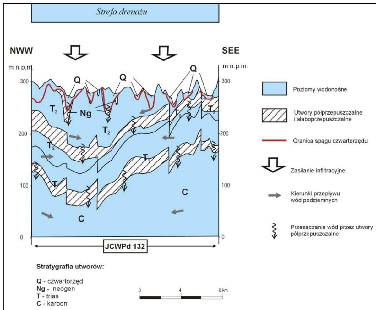
Rysunek 92. Model koncepcyjny krążenia wód podziemnych w JCWPd nr 132. Źródło: PSH
