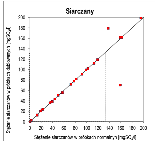
Ryc. 44. Wykres korelacji oznaczeń siarczanów w próbkach normalnych i dublowanych w zakresie stężeń 0–200 mg SO 4 /l
