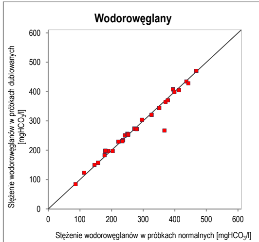
Ryc. 55. Wykres korelacji oznaczeń wodorowęglanów w próbkach normalnych i dublowanych
