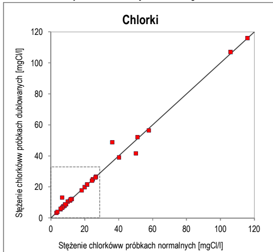
Ryc. 15. Wykres korelacji oznaczeń chlorków w próbkach normalnych i dublowanych w zakresie stężeń 0–120 mg Cl/l
