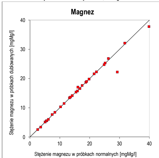
Ryc. 29. Wykres korelacji oznaczeń magnezu w próbkach normalnych i dublowanych
