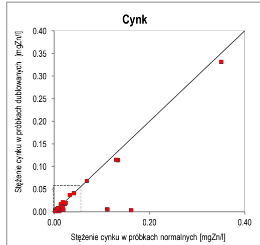
Ryc. 20. Wykres korelacji oznaczeń cynku w próbkach normalnych i dublowanych w zakresie stężeń 0–0,4 mg Zn/l
