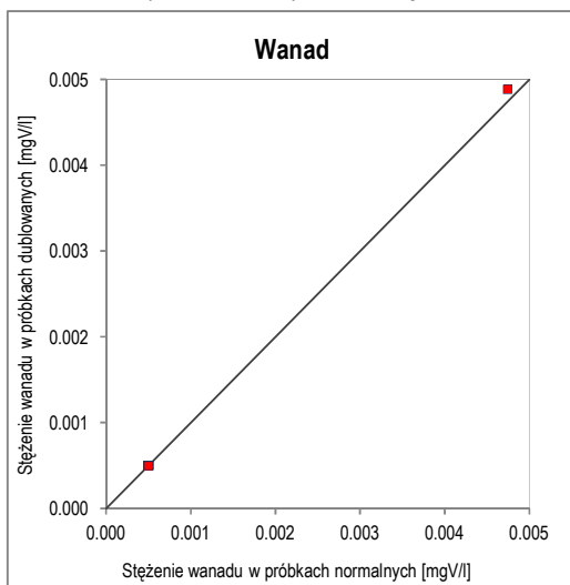
Ryc. 53. Wykres korelacji oznaczeń wanadu w próbkach normalnych i dublowanych
