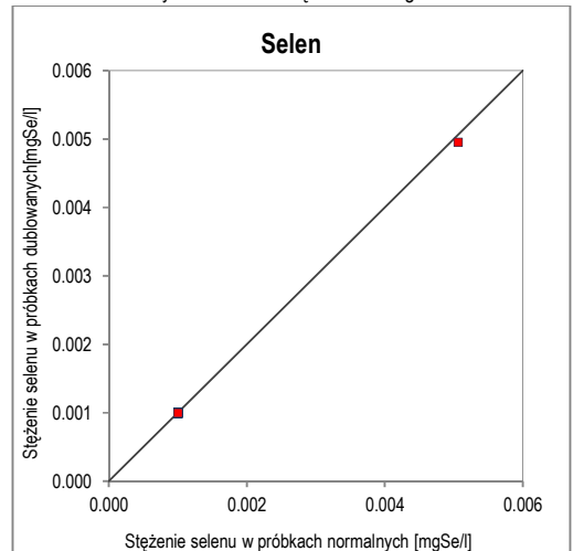
Ryc. 42. Wykres korelacji oznaczeń selenu w próbkach normalnych i dublowanych
