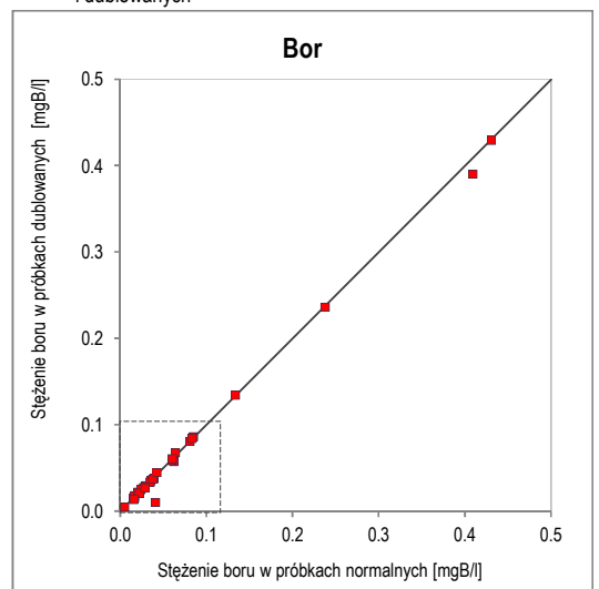
Ryc. 12. Wykres korelacji oznaczeń boru w próbkach normalnych i dublowanych w zakresie stężeń 0–0,5 mg B/l
