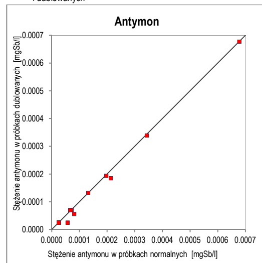
Ryc. 5. Wykres korelacji oznaczeń antymonu w próbkach normalnych i dublowanych
