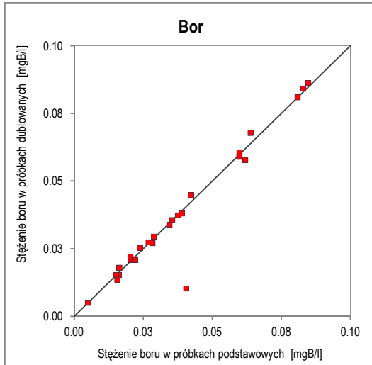
Ryc. 13. Wykres korelacji oznaczeń boru w próbkach normalnych i dublowanych w zakresie stężeń 0–0,1 mg B/l
