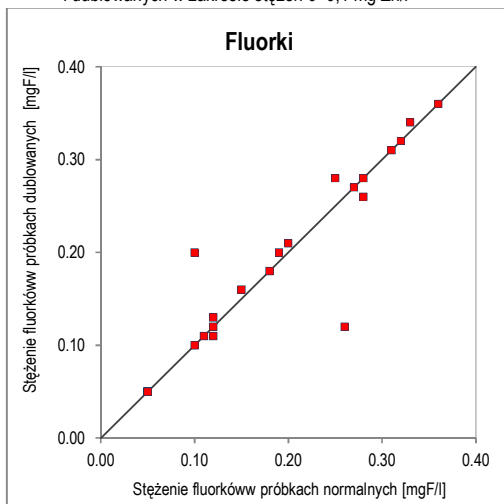
Ryc. 23. Wykres korelacji oznaczeń fluorków w próbkach normalnych i dublowanych w zakresie stężeń 0–0,4 mg F/l
