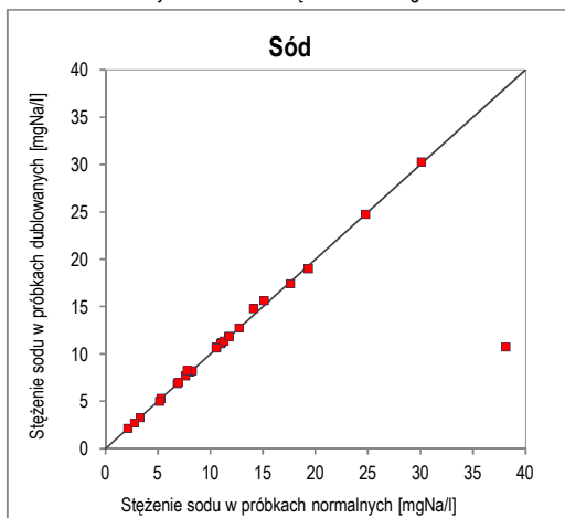
Ryc. 47. Wykres korelacji oznaczeń sodu w próbkach normalnych i dublowanych w zakresie stężeń 0–40 mg Na/l
