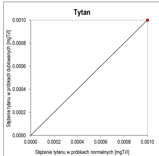
Ryc. 50. Wykres korelacji oznaczeń tytanu w próbkach normalnych i dublowanych
