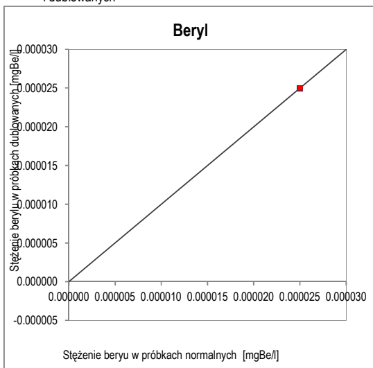
Ryc. 11. Wykres korelacji oznaczeń berylu w próbkach normalnych i dublowanych
