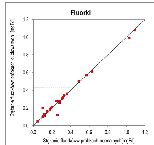
Ryc. 22. Wykres korelacji oznaczeń fluorków w próbkach normalnych i dublowanych w zakresie stężeń 0–1,2 mg F/l
