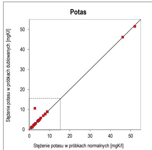
Ryc. 40. Wykres korelacji oznaczeń potasu w próbkach normalnych i dublowanych w zakresie stężeń 0–55 mg K/l
