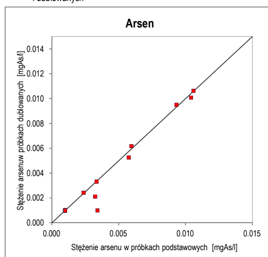
Ryc. 6. Wykres korelacji oznaczeń arsenu w próbkach normalnych i dublowanych
