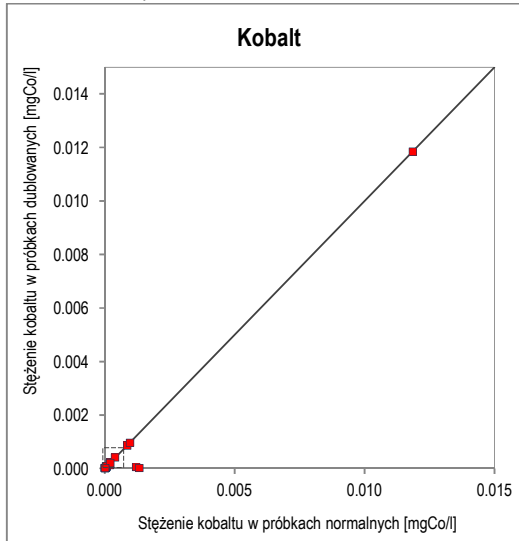
Ryc. 27. Wykres korelacji oznaczeń kobaltu w próbkach normalnych i dublowanych w zakresie stężeń 0–0,015mg Co/l
