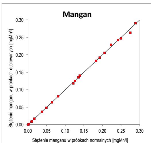
Ryc. 31. Wykres korelacji oznaczeń manganu w próbkach normalnych i dublowanych w zakresie stężeń 0–0,30 mg Mn/l
