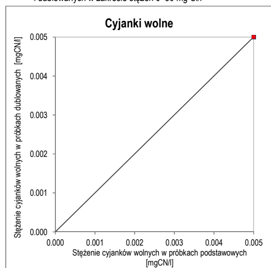
Ryc. 18. Wykres korelacji oznaczeń cyjanków wolnych w próbkach normalnych i dublowanych
