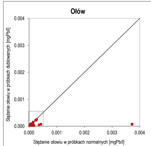
Ryc. 38. Wykres korelacji oznaczeń ołowiu w próbkach normalnych i dublowanych w zakresie stężeń 0–0,004 mg Pb/l
