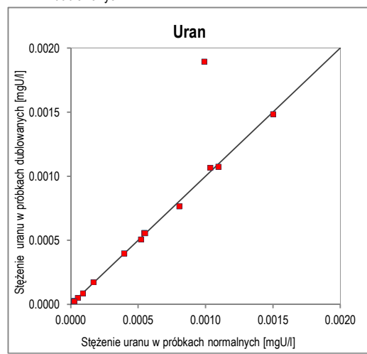
Ryc. 52. Wykres korelacji oznaczeń uranu w próbkach normalnych i dublowanych w zakresie stężeń 0–0,002 mg U/l
