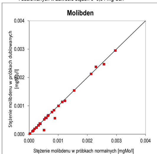
Ryc. 35. Wykres korelacji oznaczeń molibdenu w próbkach normalnych i dublowanych w zakresie stężeń 0–0,004 mg Mo/l
