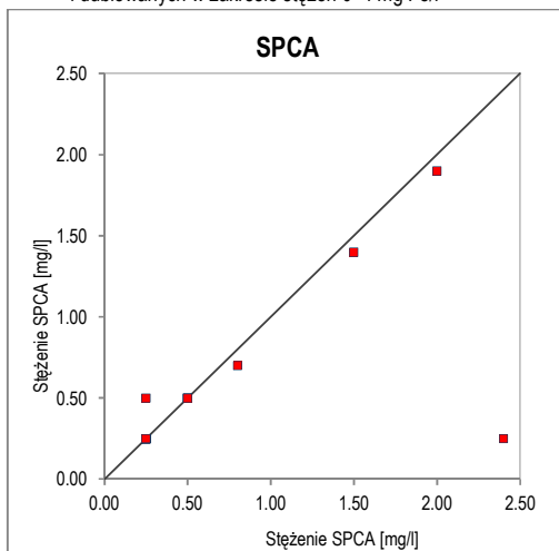
Ryc. 59. Wykres korelacji oznaczeń SPCA w próbkach normalnych i dublowanych w zakresie stężeń 0–2.50 mg SPCA/l
