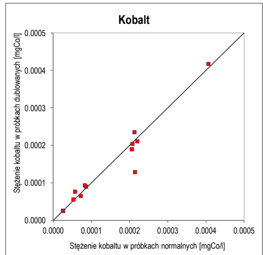
Ryc. 28. Wykres korelacji oznaczeń kobaltu w próbkach normalnych i dublowanych w zakresie stężeń 0–0,0005mg Co/l
