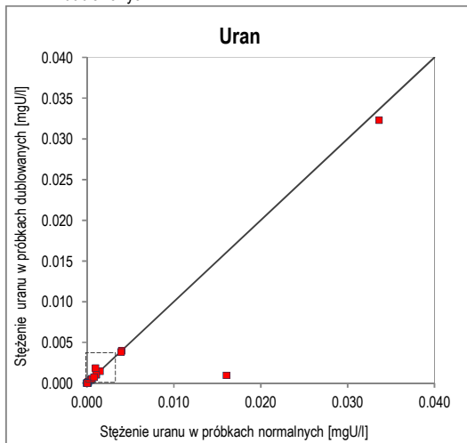
Ryc. 51. Wykres korelacji oznaczeń uranu w próbkach normalnych i dublowanych w zakresie stężeń 0–0,04 mg U/l
