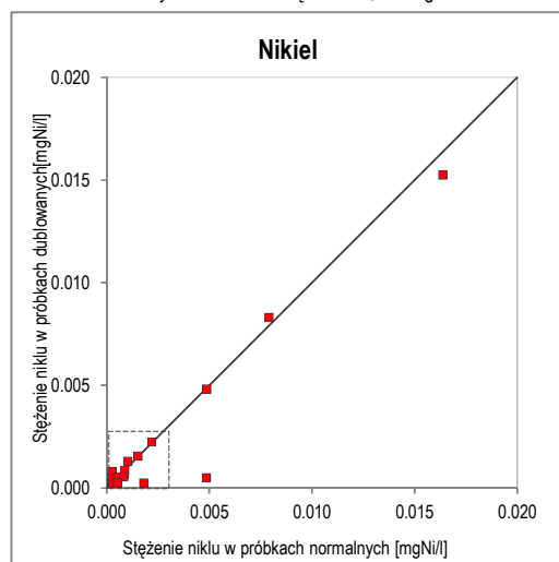
Ryc. 36. Wykres korelacji oznaczeń niklu w próbkach normalnych i dublowanych w zakresie stężeń 0–0,020 mg Ni/l
