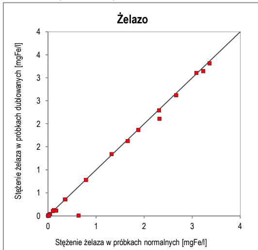
Ryc. 57. Wykres korelacji oznaczeń żelaza w próbkach normalnych i dublowanych w zakresie stężeń 0–4 mg Fe/l
