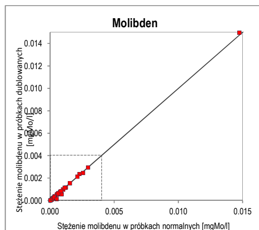
Ryc. 34. Wykres korelacji oznaczeń molibdenu w próbkach normalnych i dublowanych w zakresie stężeń 0–0,015 mg Mo/l
