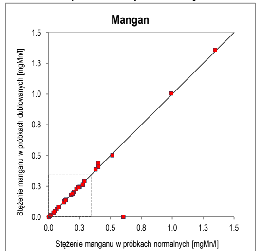
Ryc. 30. Wykres korelacji oznaczeń manganu w próbkach normalnych i dublowanych w zakresie stężeń 0–1,15 mg Mn/l
