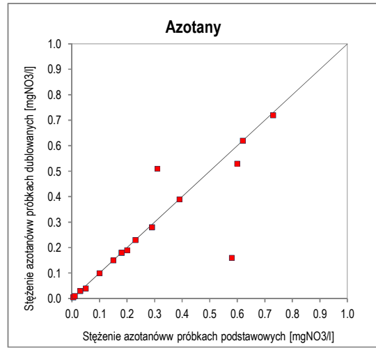
Ryc. 8. Wykres korelacji oznaczeń azotanów w próbkach normalnych i dublowanych w zakresie stężeń 0–1 mg NO 3 /l
