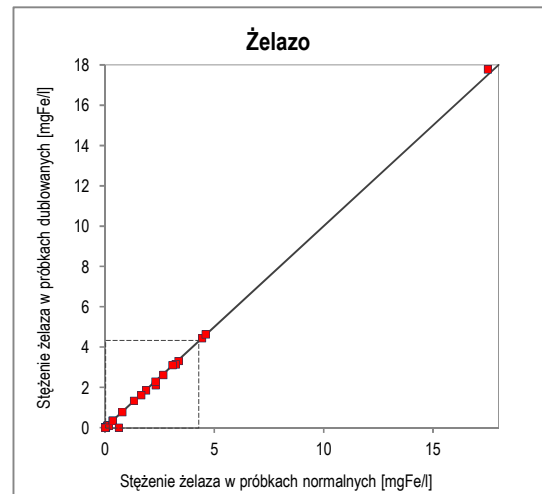
Ryc. 56. Wykres korelacji oznaczeń żelaza w próbkach normalnych i dublowanych w zakresie stężeń 0–18 mg Fe/l
