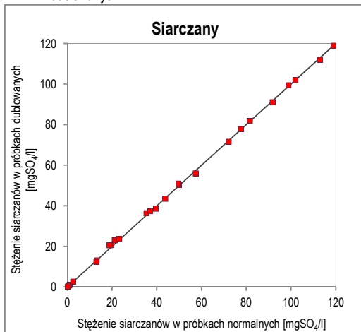
Ryc. 45. Wykres korelacji oznaczeń siarczanów w próbkach normalnych i dublowanych w zakresie stężeń 0–120 mg SO 4 /l
