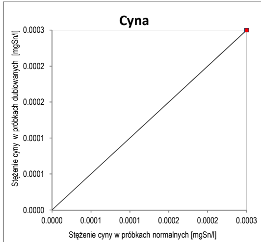
Ryc. 19. Wykres korelacji oznaczeń cyny w próbkach normalnych i dublowanych
