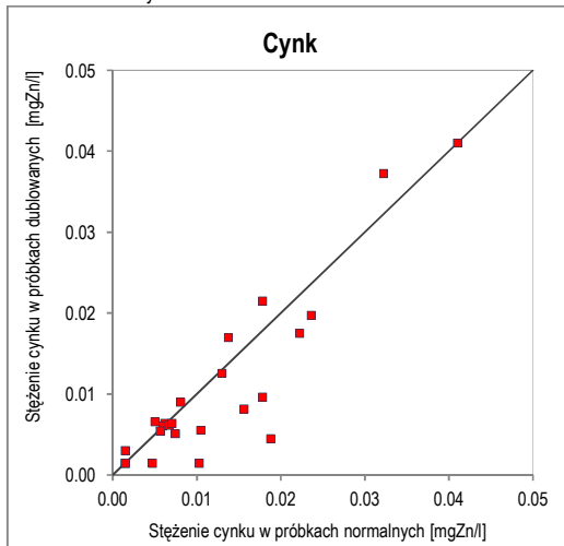
Ryc. 21. Wykres korelacji oznaczeń cynku w próbkach normalnych i dublowanych w zakresie stężeń 0–0,4 mg Zn/l
