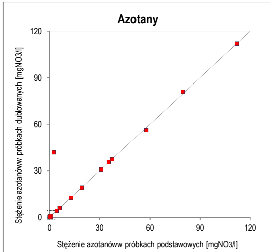
Ryc. 7. Wykres korelacji oznaczeń azotanów w próbkach normalnych i dublowanych w zakresie stężeń 0–120 mg NO 3 /l
