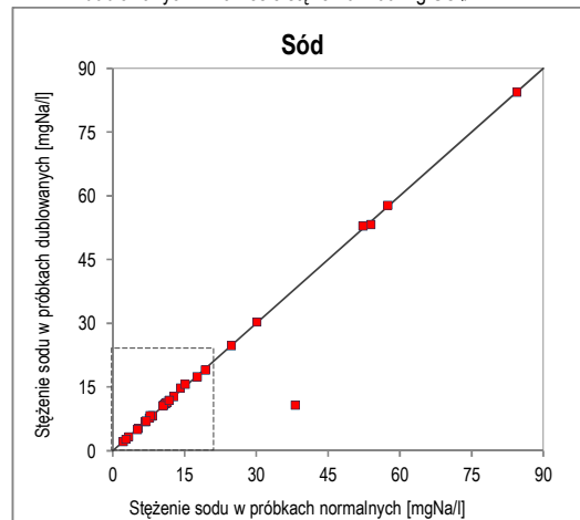
Ryc. 46. Wykres korelacji oznaczeń sodu w próbkach normalnych i dublowanych w zakresie stężeń 0–15 mg Na/l
