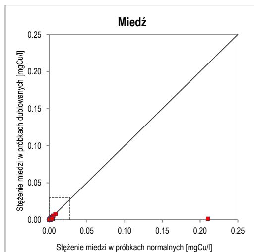
Ryc. 32. Wykres korelacji oznaczeń miedzi w próbkach normalnych i dublowanych w zakresie stężeń 0–2,5 mg Cu/l
