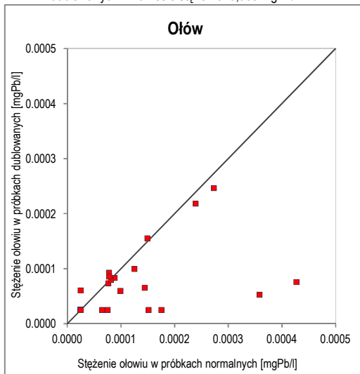
Ryc. 39. Wykres korelacji oznaczeń ołowiu w próbkach normalnych i dublowanych w zakresie stężeń 0–0,0005 mg Pb/l
