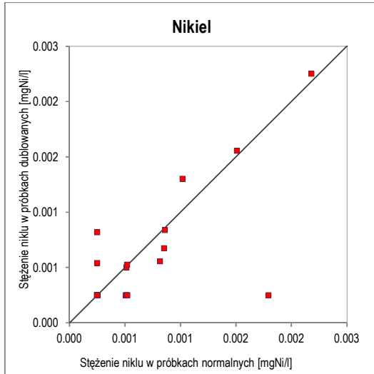
Ryc. 37. Wykres korelacji oznaczeń niklu w próbkach normalnych i dublowanych w zakresie stężeń 0–0,003 mg Ni/l
