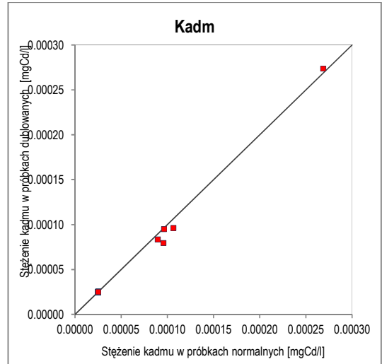
Ryc. 26. Wykres korelacji oznaczeń kadmu w próbkach normalnych i dublowanych
