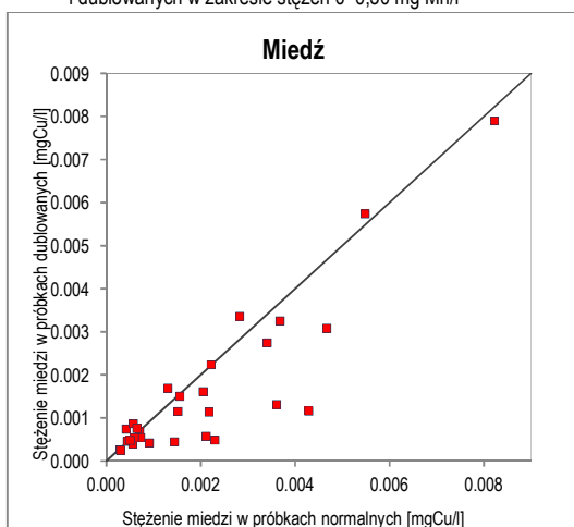
Ryc. 33. Wykres korelacji oznaczeń miedzi w próbkach normalnych i dublowanych w zakresie stężeń 0–0,01 mg Cu/l
