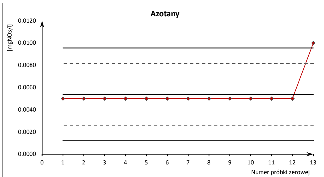
Ryc. 1. Karta kontrolna pojedynczych pomiarów oznaczeń azotanów
