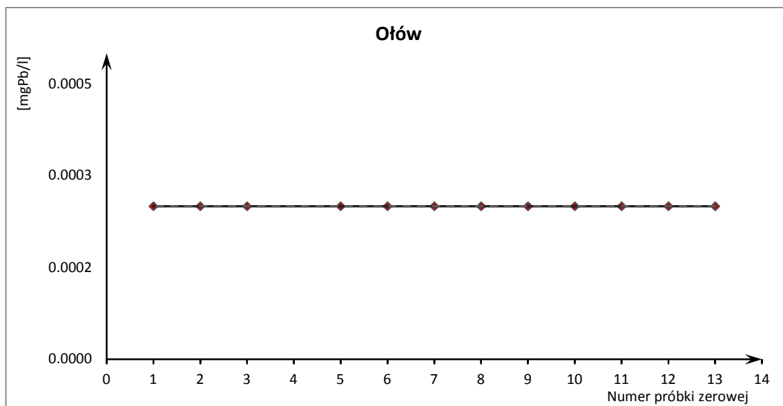
Ryc. 18. Karta kontrolna pojedynczych pomiarów oznaczeń ołowiu po wyłączeniu sygnałów punktowych
