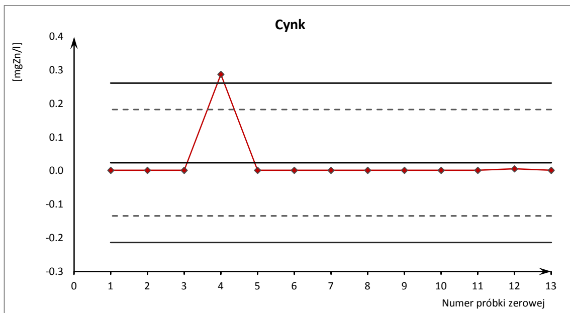
Ryc. 8. Karta kontrolna pojedynczych pomiarów oznaczeń cynku
