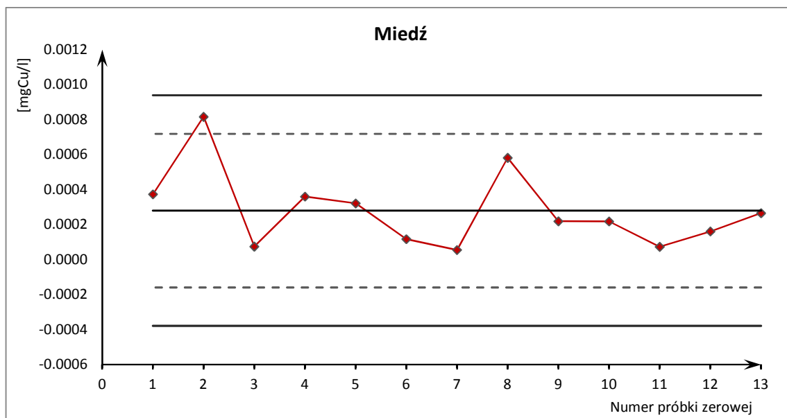
Ryc. 16. Karta kontrolna pojedynczych pomiarów oznaczeń miedzi
