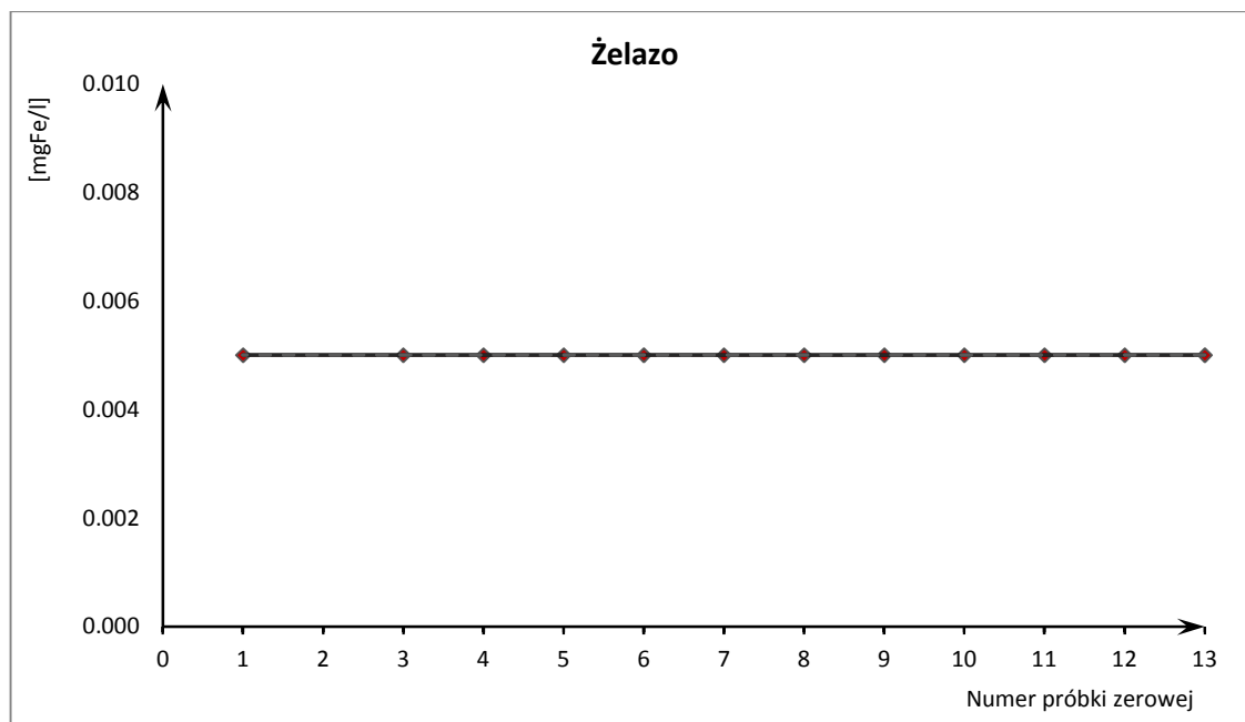
Ryc. 23. Karta kontrolna pojedynczych pomiarów oznaczeń żelaza po wyłączeniu sygnałów punktowych
