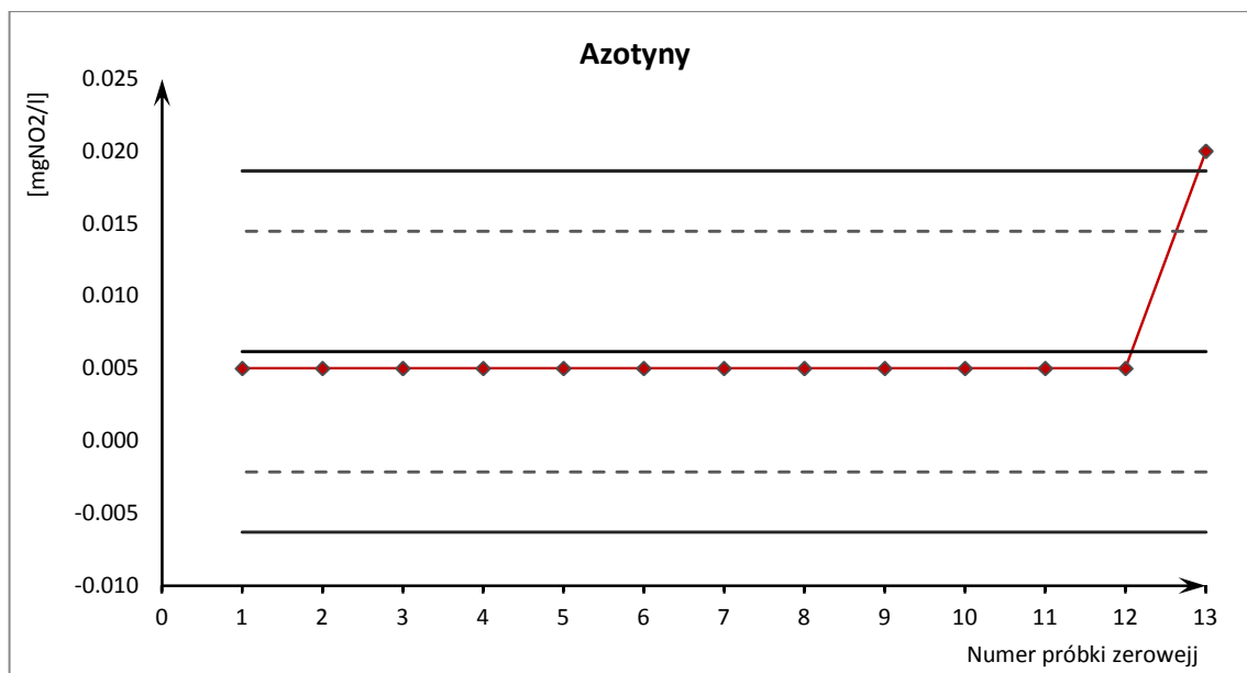
Ryc. 3. Karta kontrolna pojedynczych pomiarów oznaczeń azotynów
