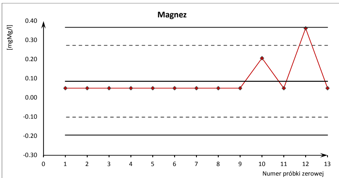
Ryc. 14. Karta kontrolna pojedynczych pomiarów oznaczeń magnezu
