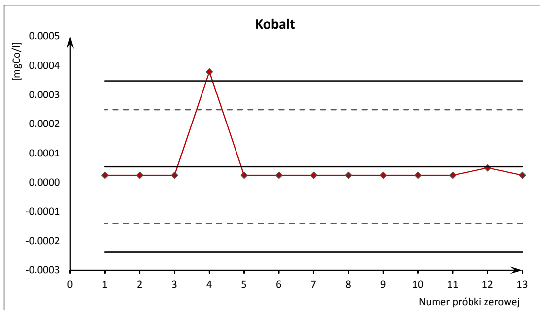
Ryc. 12. Karta kontrolna pojedynczych pomiarów oznaczeń kobaltu
