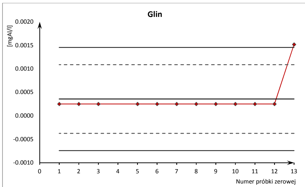
Ryc. 11. Karta kontrolna pojedynczych pomiarów oznaczeń glinu po wyłączeniu sygnałów punktowych
