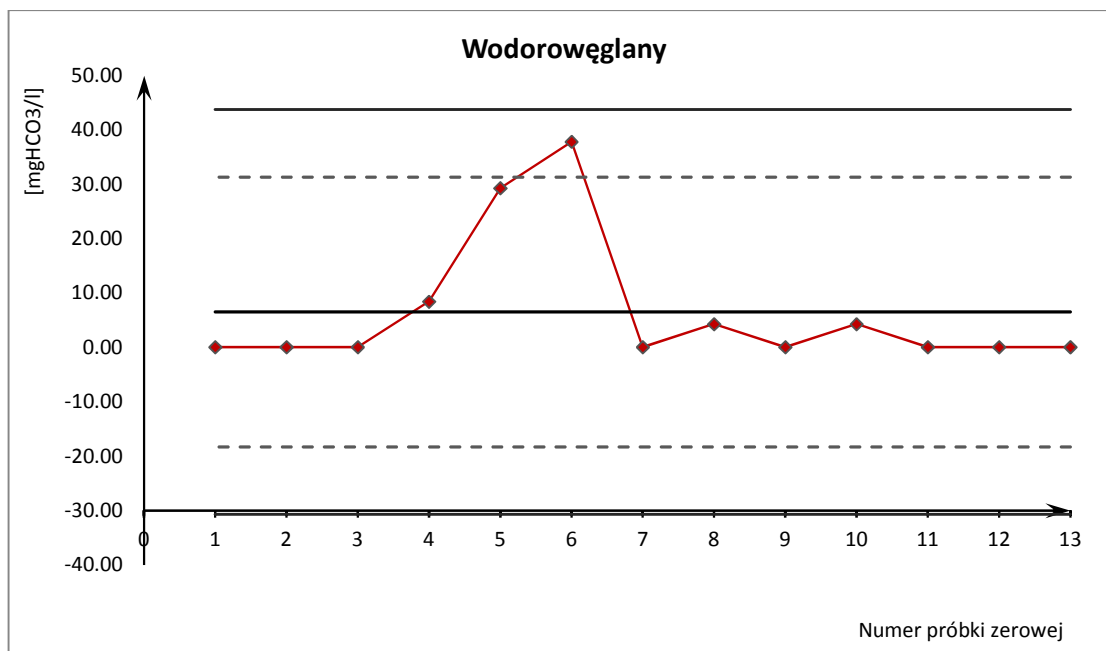
Ryc. 21. Karta kontrolna pojedynczych pomiarów oznaczeń wodorowęglanów
