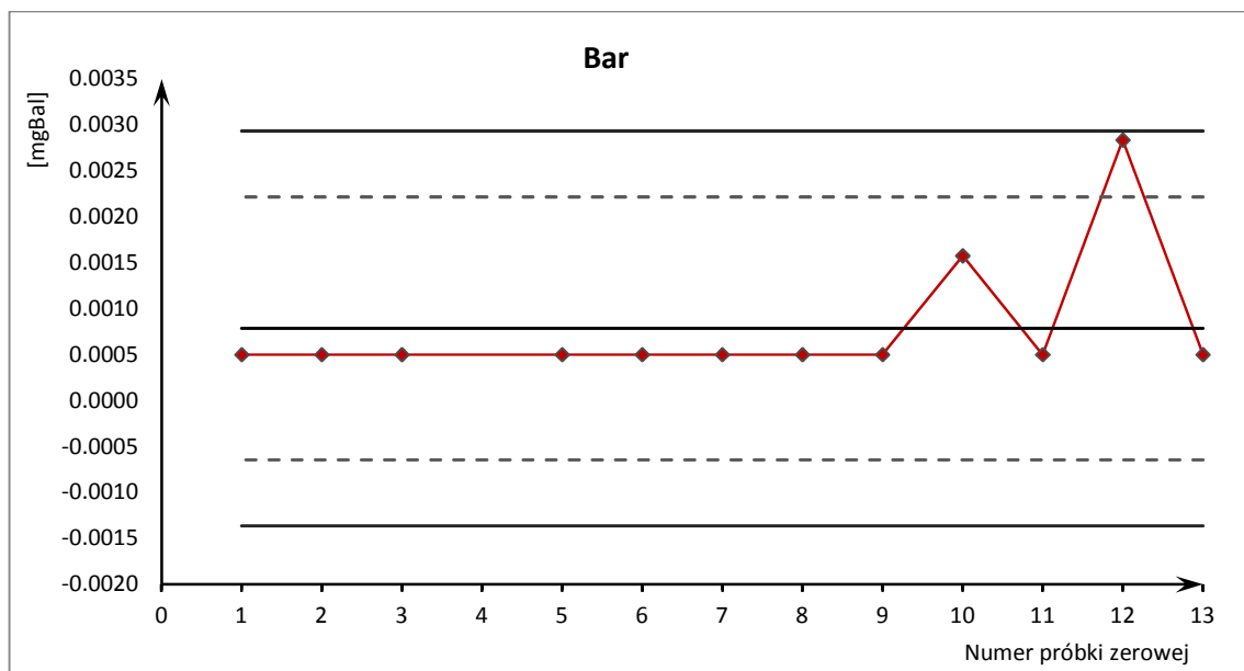
Ryc. 6 . Karta kontrolna pojedynczych pomiarów oznaczeń baru po wyłączeniu sygnałów punktowych
