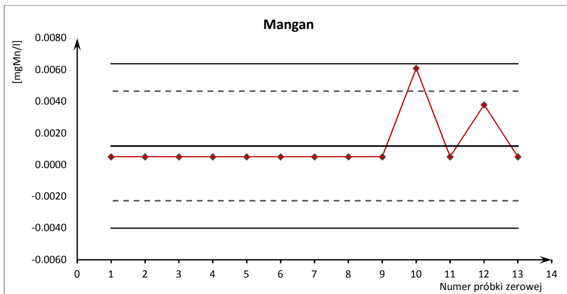
Ryc. 15. Karta kontrolna pojedynczych pomiarów oznaczeń manganu
