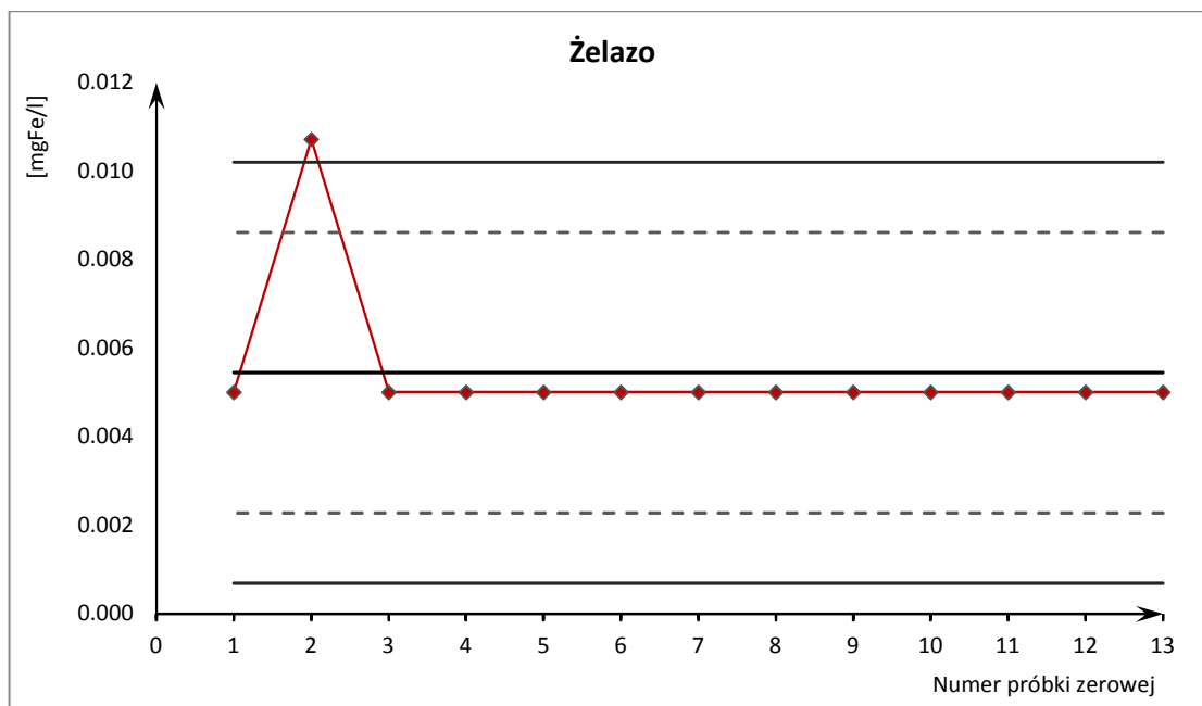
Ryc. 22. Karta kontrolna pojedynczych pomiarów oznaczeń żelaza
