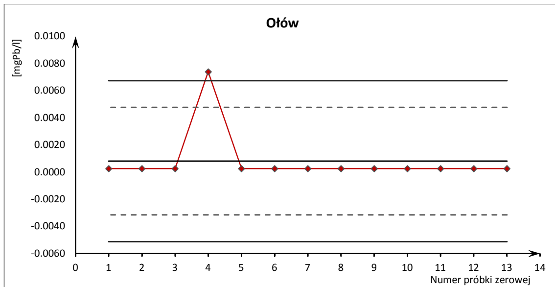
Ryc. 17. Karta kontrolna pojedynczych pomiarów oznaczeń ołowiu
