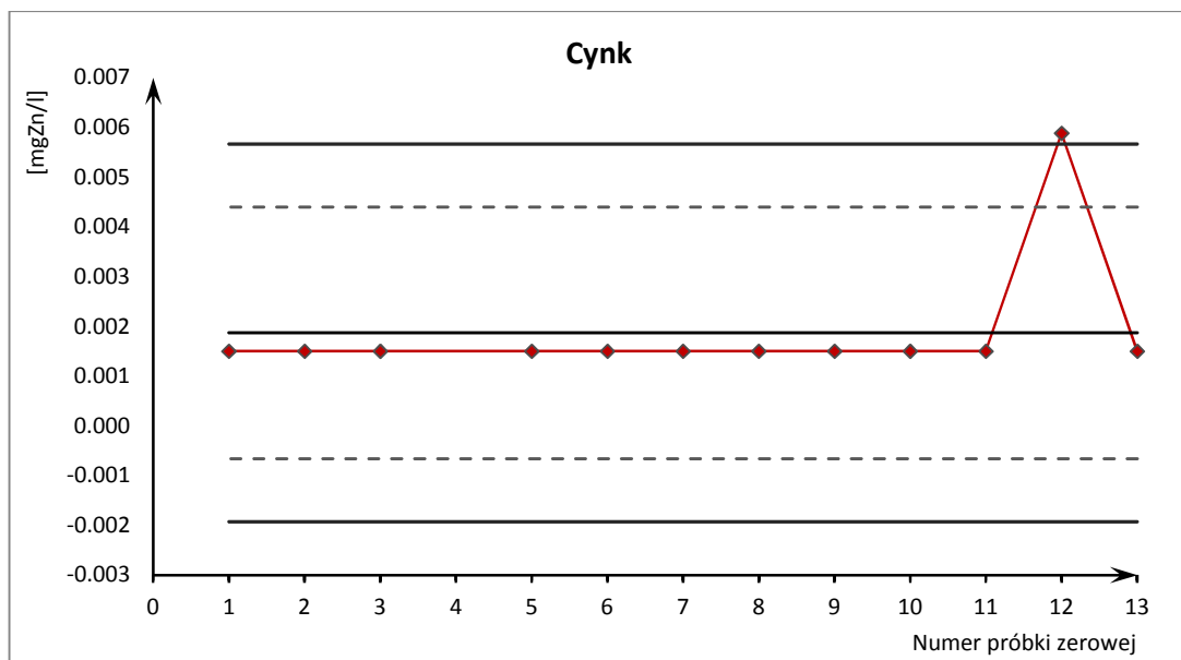
Ryc. 9. Karta kontrolna pojedynczych pomiarów oznaczeń cynku po wyłączeniu sygnałów punktowych
