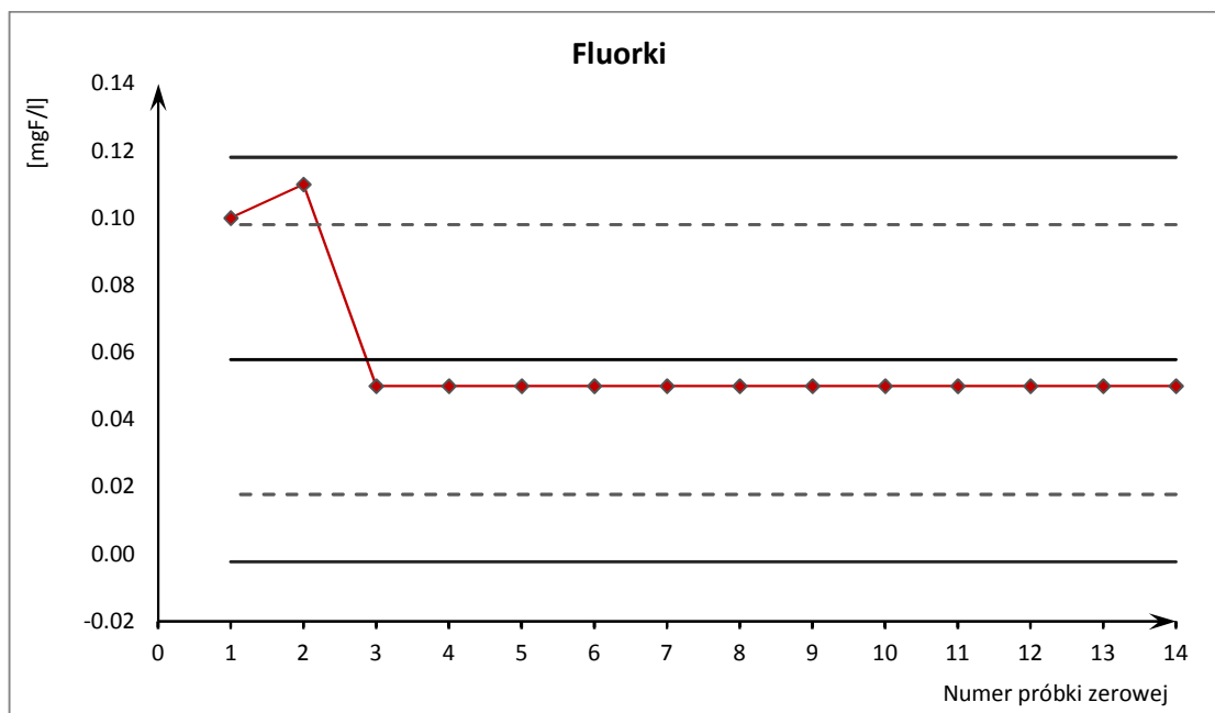
Ryc. 20. Karta kontrolna pojedynczych pomiarów oznaczeń fluorków
