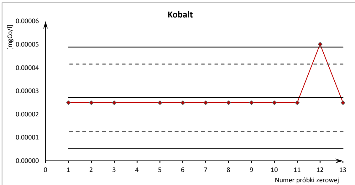
Ryc. 13. Karta kontrolna pojedynczych pomiarów oznaczeń kobaltu po wyłączeniu sygnałów punktowych
