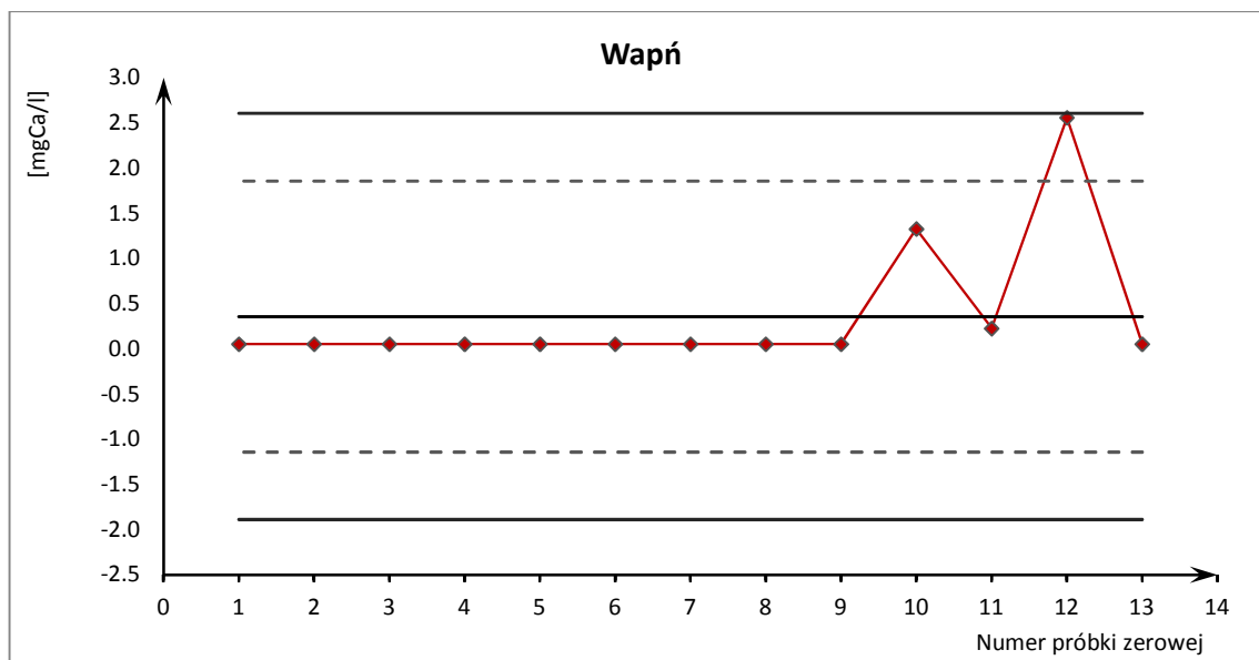
Ryc. 19. Karta kontrolna pojedynczych pomiarów oznaczeń wapnia
