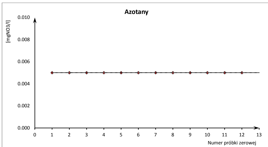
Ryc. 2. Karta kontrolna pojedynczych pomiarów oznaczeń azotanów po wyłączeniu sygnałów punktowych
