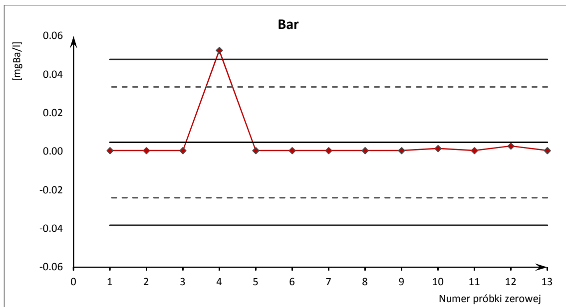
Ryc. 5. Karta kontrolna pojedynczych pomiarów oznaczeń baru
