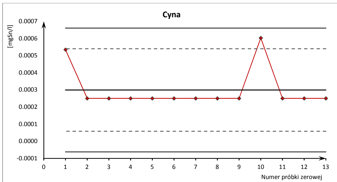
Ryc. 7. Karta kontrolna pojedynczych pomiarów oznaczeń cyny
