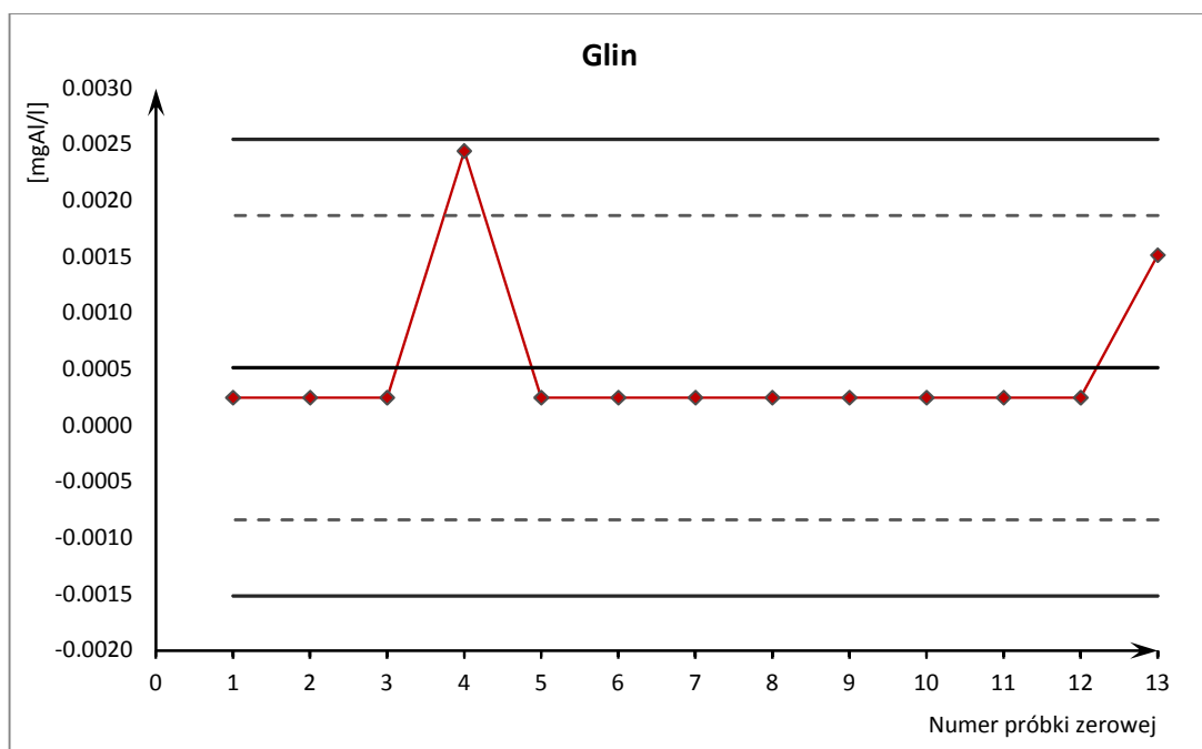
Ryc. 10. Karta kontrolna pojedynczych pomiarów oznaczeń glinu
